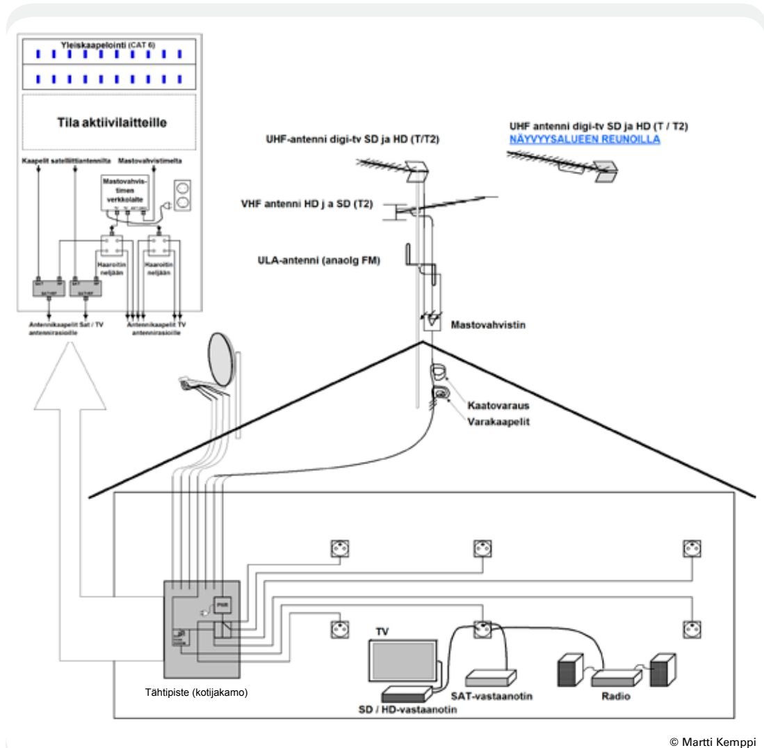
Pientalon antennijärjestelmä.
