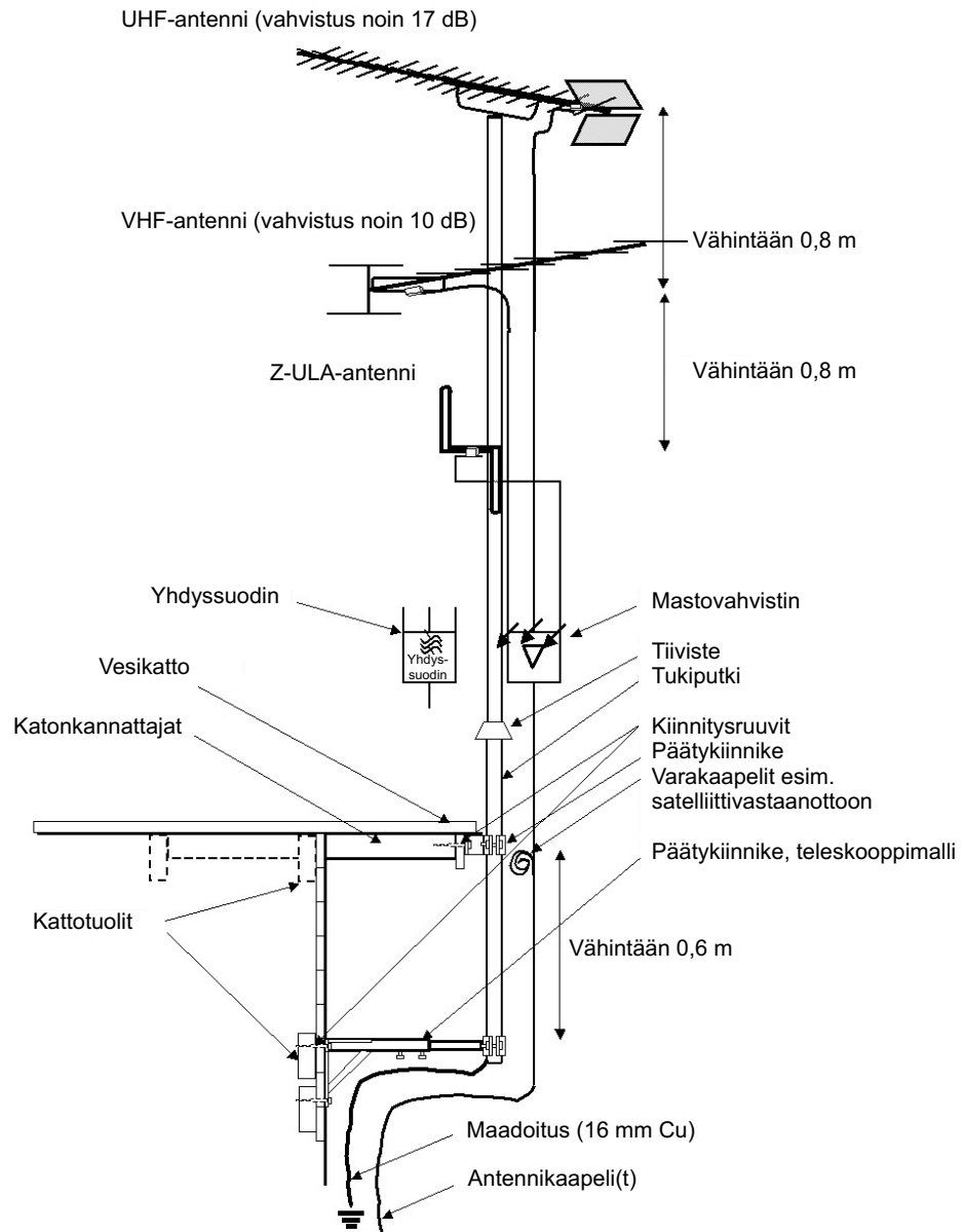
Antennimaston ja antennien asennus rakennuksen pätyyn.
